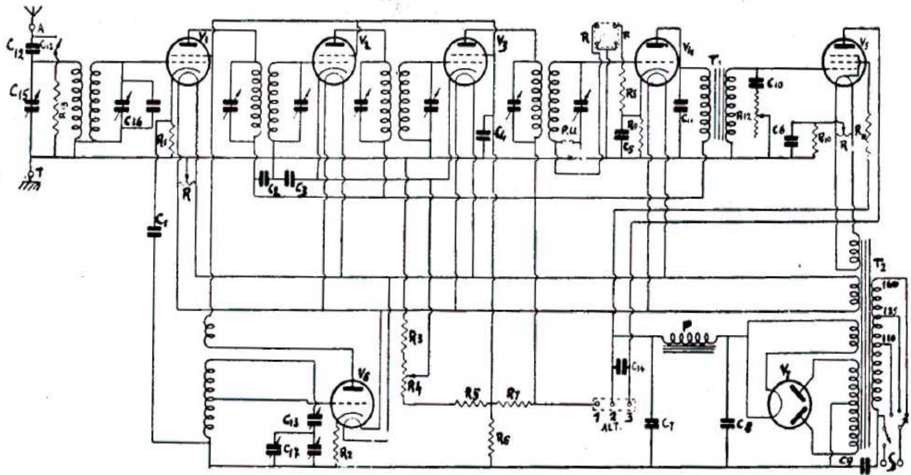
Allochio Bacchini F61 CA
